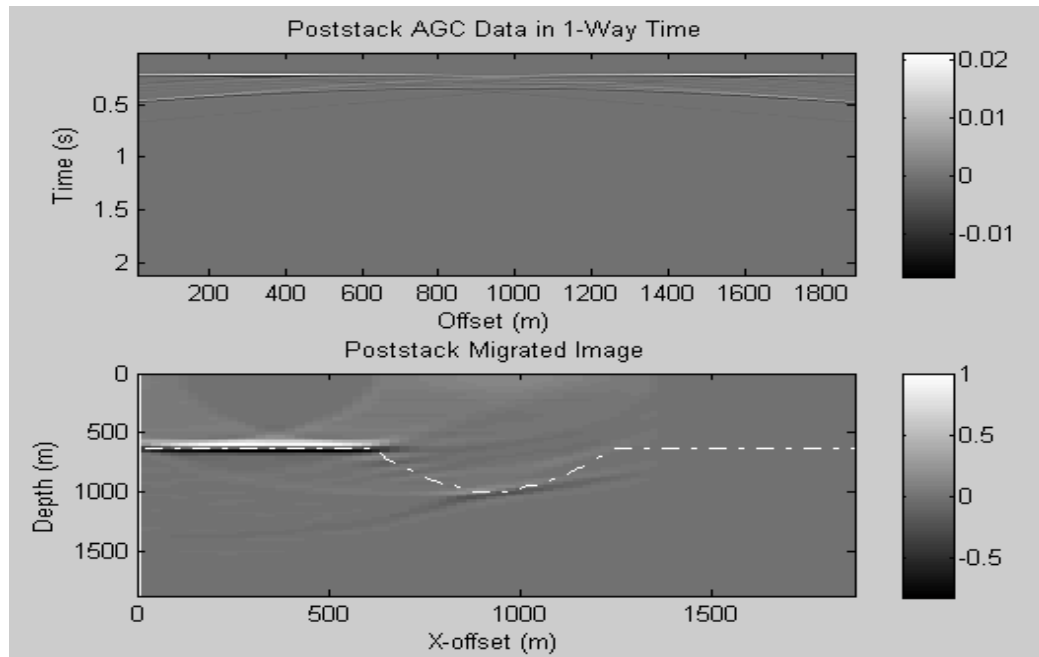
附图4 叠后（上）与叠后偏移（下）地震剖面
